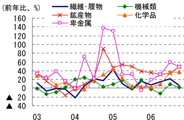
（図表 3） 輸出
